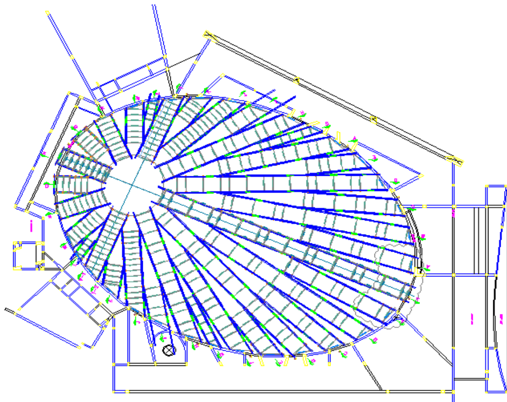
Vista en planta del sistema de andamiaje diseñado por Ulma.
