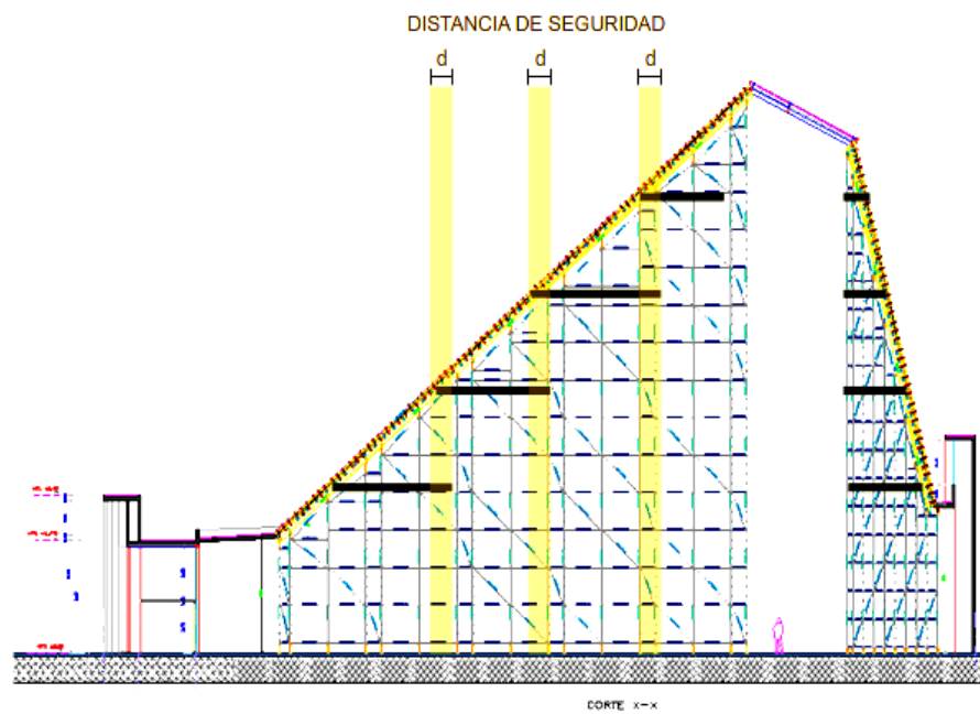
Vista en corte de la implementación de mallas de seguridad y plataformas de trabajo interior
