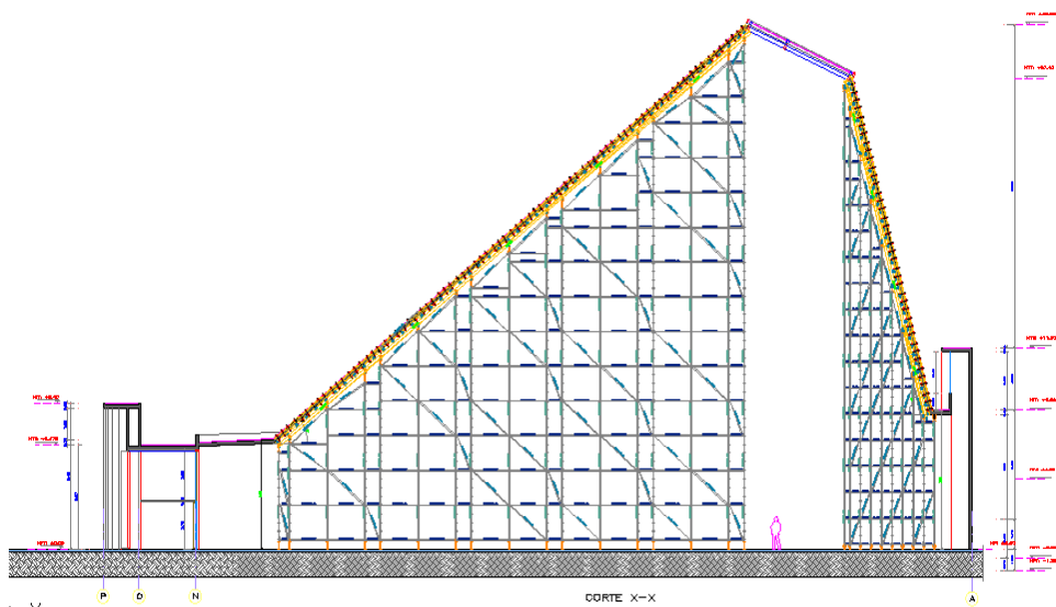
Vista en corte de la estructura del soporte de encofrado. No figura la escalera metálica de acceso interior, la cual estuvo ubicada en el espacio en blanco (debajo de la cima de la cúpula)
