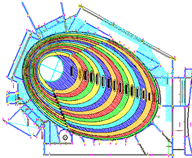
Vista en planta de los sectores de vaciado (semianillos)
