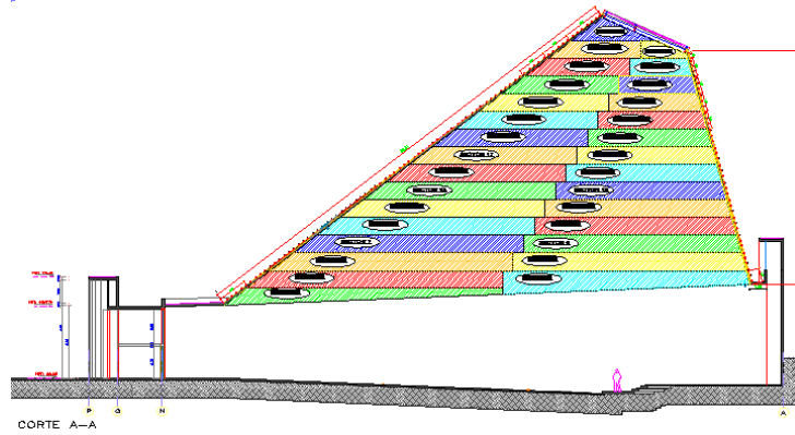
Vista en corte de los sectores de vaciado (semianillos)
