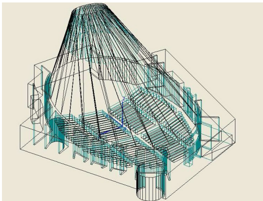
Imágenes de conceptualización de la geometría de la cúpula en 3D
