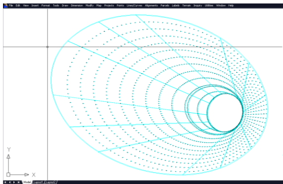
Vista de curvas de nivel de la cúpula y las cotas de referencia en el modelo 3D.
