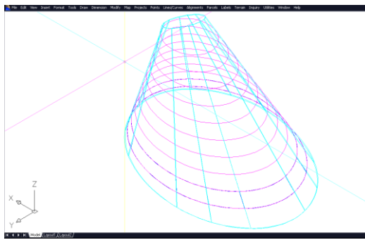
Secciones horizontales de vaciado de cúpula plasmado en el modelo 3D.
